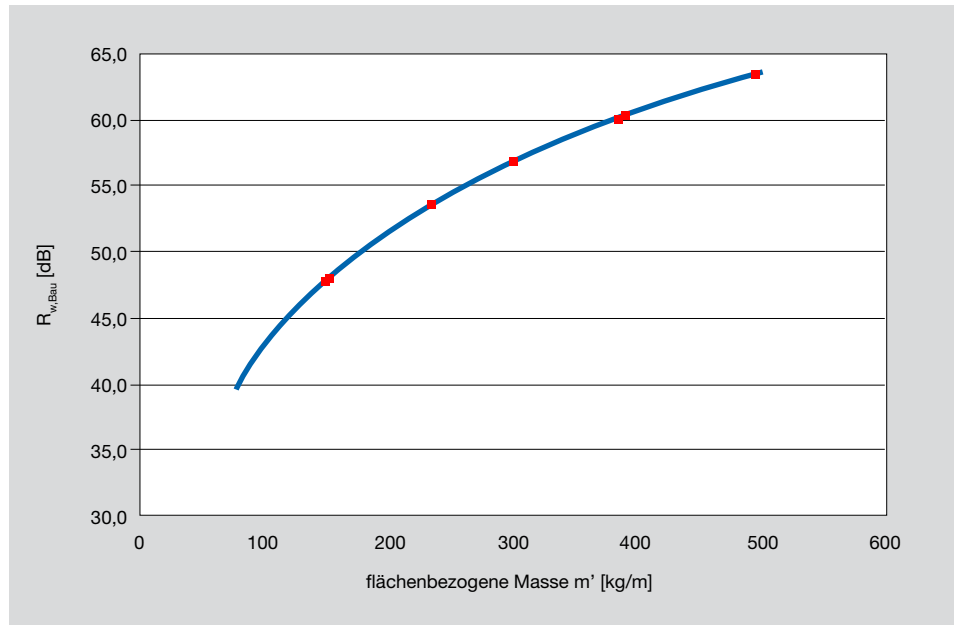
Bild 3: Massekurve für Mauerwerk aus Leichtbetonsteinen
