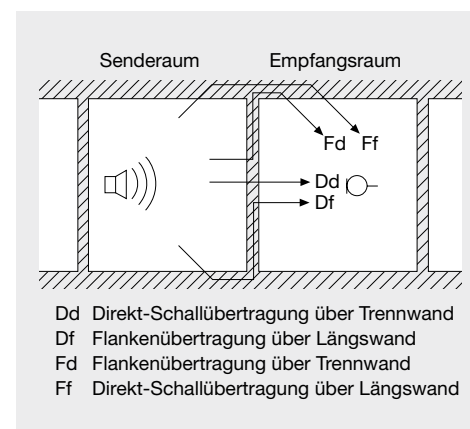
Bild 2: Schallübertragung zwischen dem lauten Senderraum und dem leisen Empfangsraum über das trennende Bauteil und die flankierenden Bauteile
