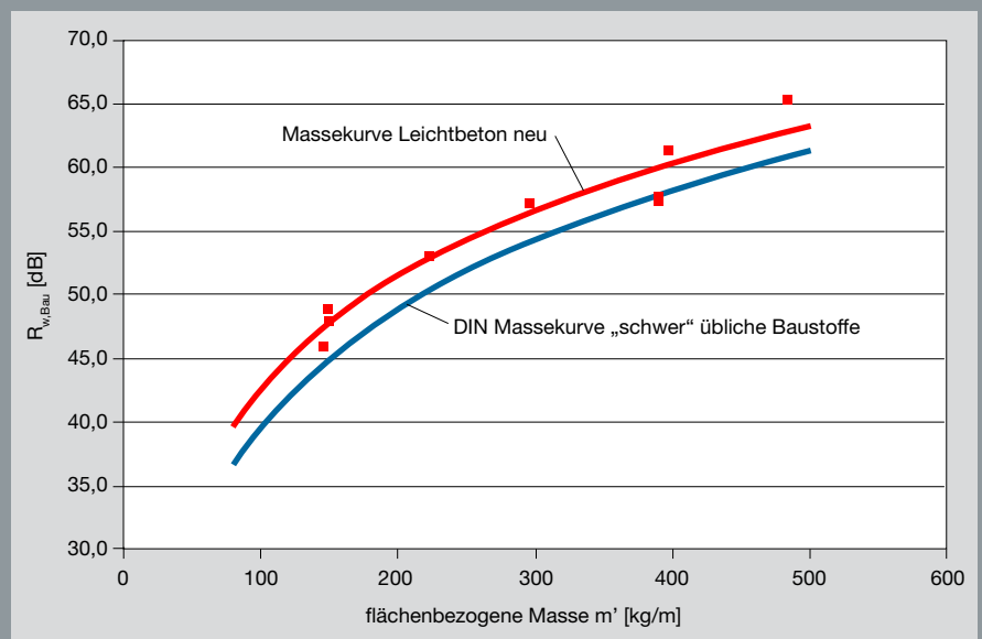
Bild 1: Massekurve Entwurf DIN 4109
