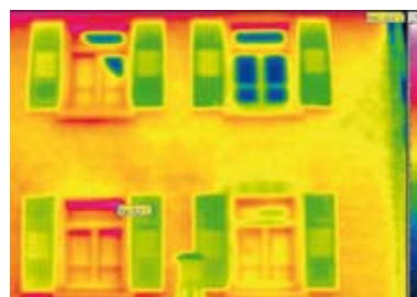
1b: Thermografieaufnahme
